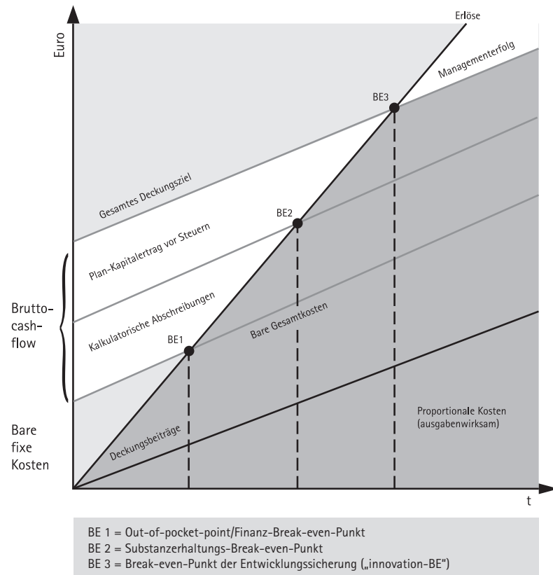
Abb. 6: Break-even-Diagramm mit Zwischenzielen 7
